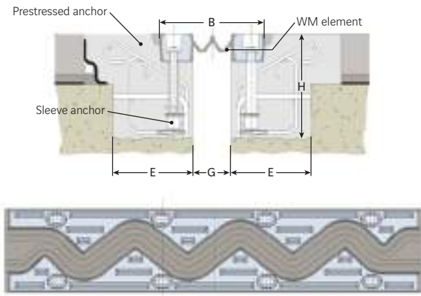
WM 80
