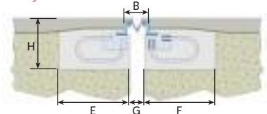
Freyssimod LW 80
