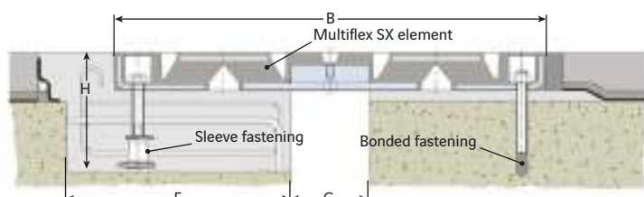
Double element module
